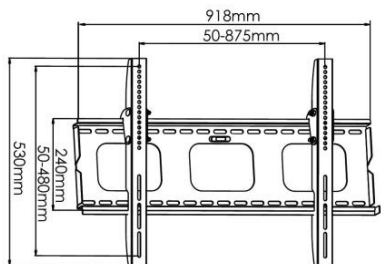
012-1024 Supporto a parete fisso 42"-86" Antifurto
