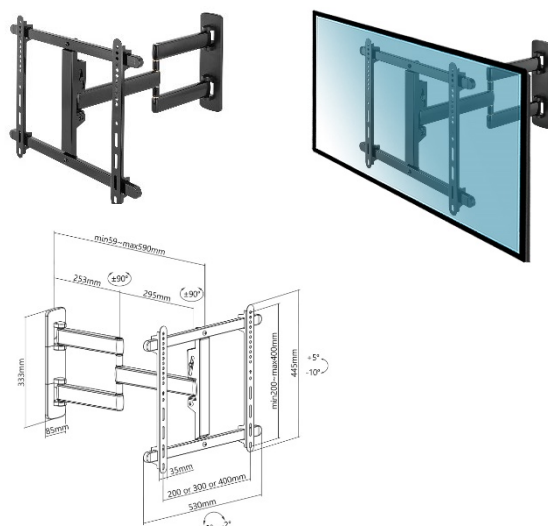
013-3145 Supporto a parete snodabile Pro 32"-55"
