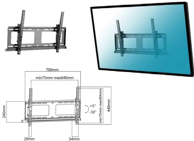
012-1364 Supporto inclinabile 37"-75" Antifurto
