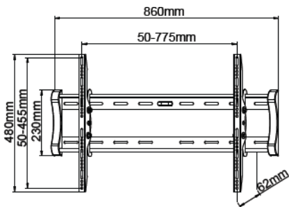
012-1243 Supporto a parete inclinabile 32"-60"
