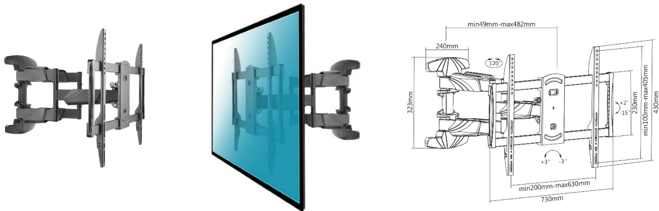
013-2664 Supporto a parete orientabile inclinabile 37''-70''
