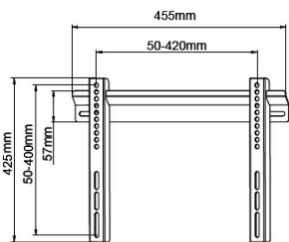
012-1142 Supporto a parete fisso 23"-55"
