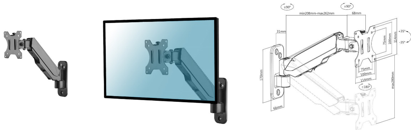
016-1511 Supporto a parete ultra-regolabile per schermi e monitor 17"-32"
