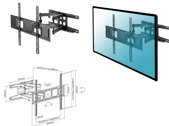
013-3145 Supporto a parete snodabile Pro 32"-55"
