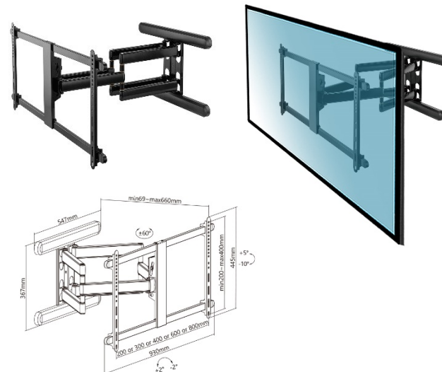
013-3245 Supporto a parete snodabile Pro 43"-90"
