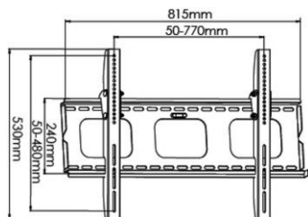
012-1023 Supporto a parete fisso 32"-60" Antifurto
