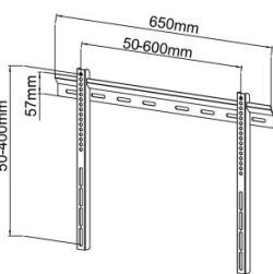
012-1143 Supporto a parete fisso 32"-60"
