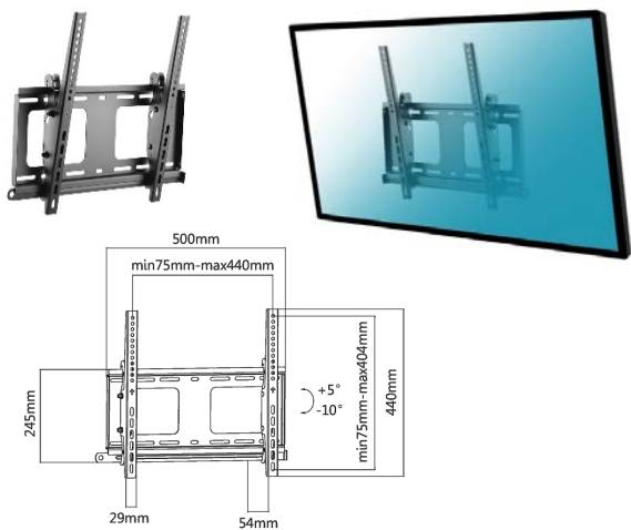
012-1344 Supporto inclinabile 32"-55" Antifurto
