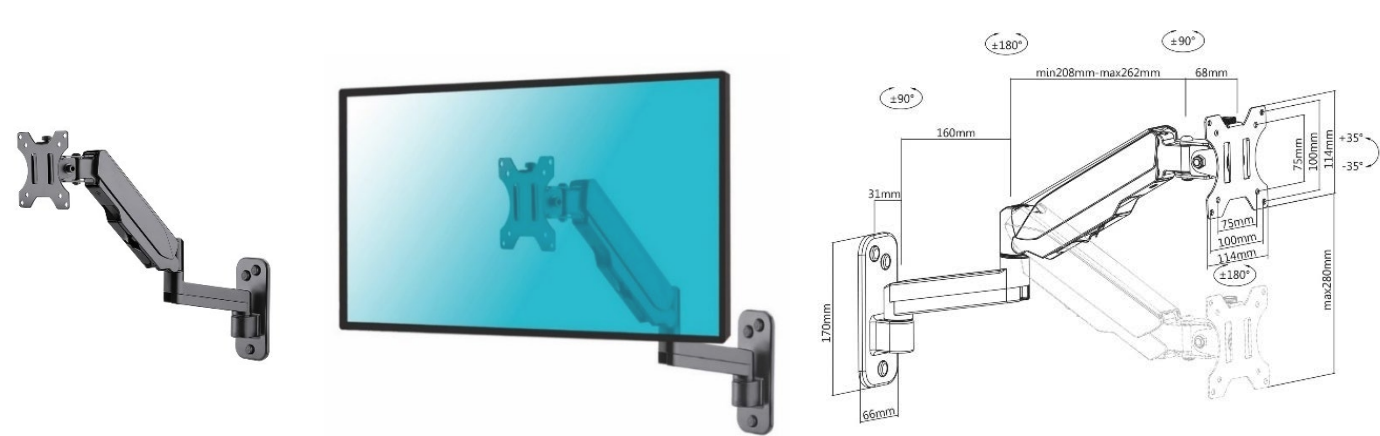
016-1501 Supporto a parete ultra-regolabile per schermi e monitor 17"-32"
