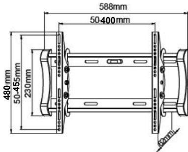
012-1242 Supporto a parete inclinabile 23"-55"
