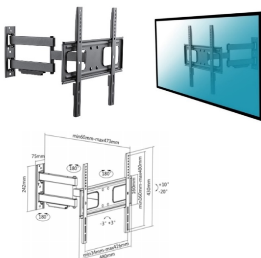
013-3245 Supporto a parete snodabile Pro 43"-90"
