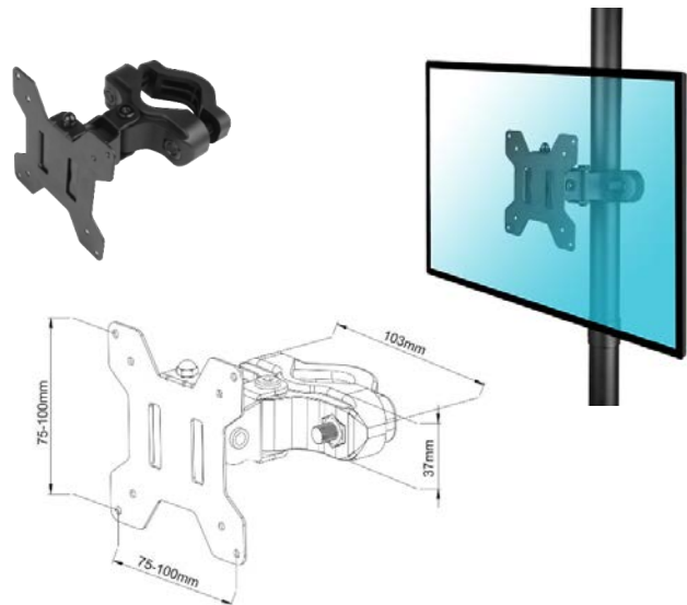
018-1311 Supporto snodabile per struttura TRUSS 13"-30" Compatibilità tubi : 28 à 60 mm
