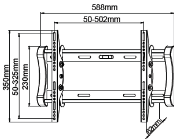
012-1241 Supporto a parete inclinabile 23"-37"
