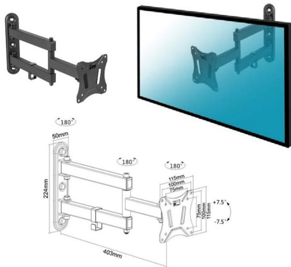
013-1121 Supporto a parete orientabile inclinabile 13"-27" Doppio braccio
