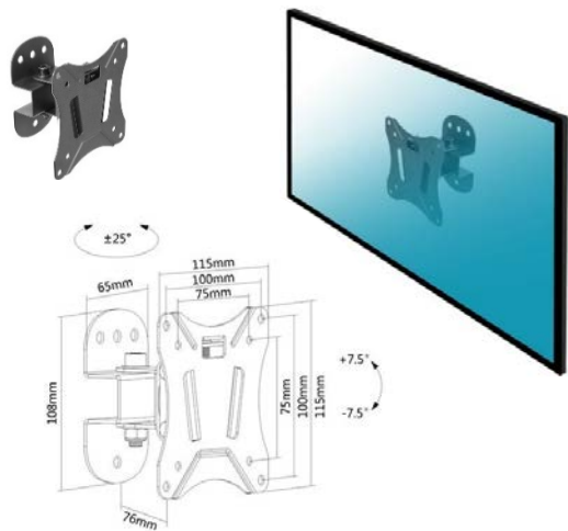
013-1101 Supporto a parete orientabile inclinabile 13"-27"
