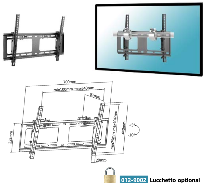
018-1364 Supporto inclinabile per struttura TRUSS 37"-75" Compatibilità tube : 48 à 51 mm
