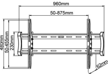
012-1244 Supporto a parete inclinabile 42"-75"
