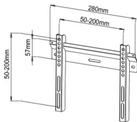
012-1140 Supporto a parete fisso 19"-37"
