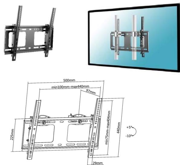
018-1344 Supporto inclinabile per struttura TRUSS 32"-55" Compatibilità tube : 48 à 51 mm
