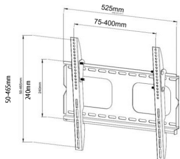
012-1022 Supporto a parete fisso 23"-55" Antifurto
