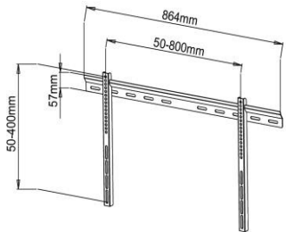
012-1144 Supporto a parete fisso 42"-70"
