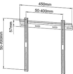
012-1141 Supporto a parete fisso 23"-37"
