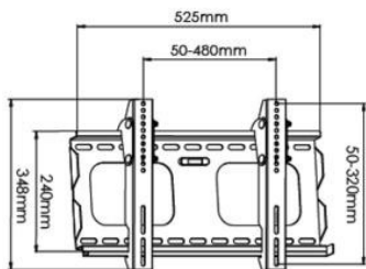
012-1021 Supporto a parete fisso 23"-37" Antifurto
