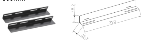
110-0185 Kit 2 rails Lunghezza 320mm Compatibile rack 112-66 de profondità 600mm
