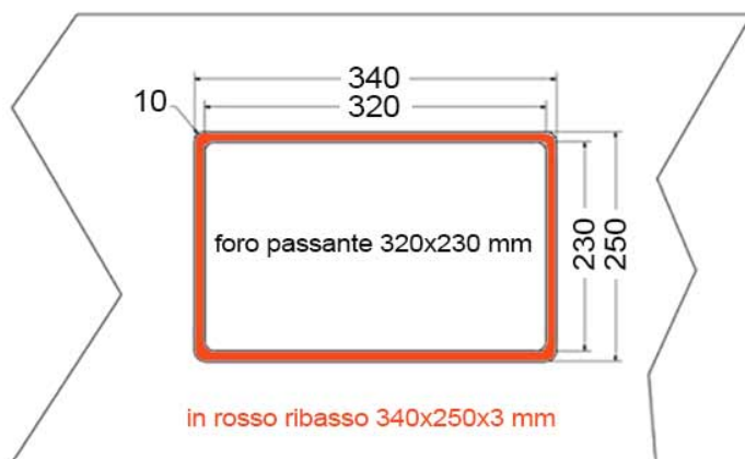
Piano di alloggiamento
